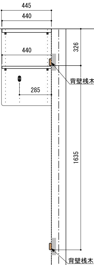
A-A' 断面
