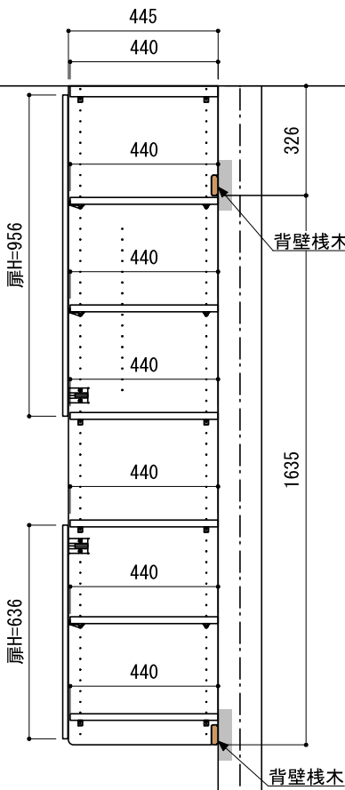
B-B' 断面
