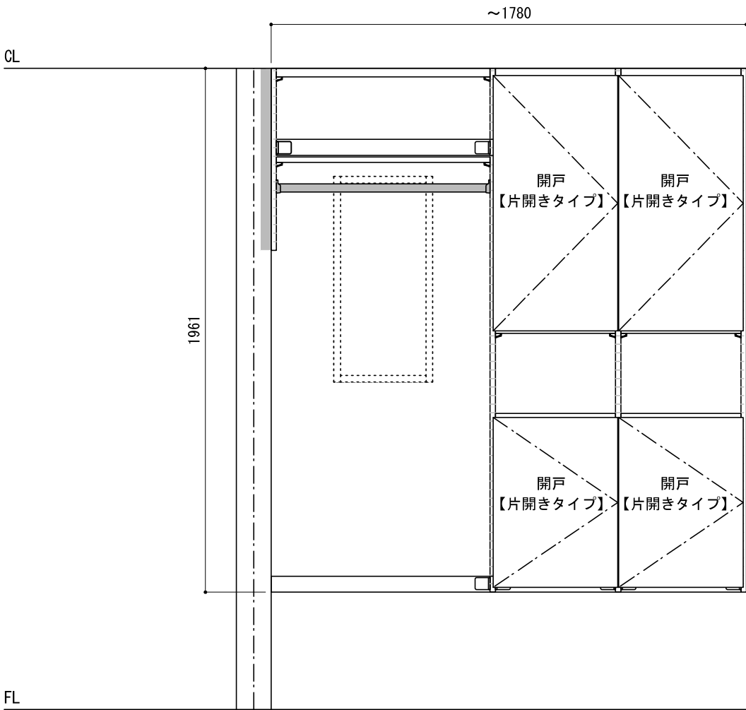
正面図（外観）
