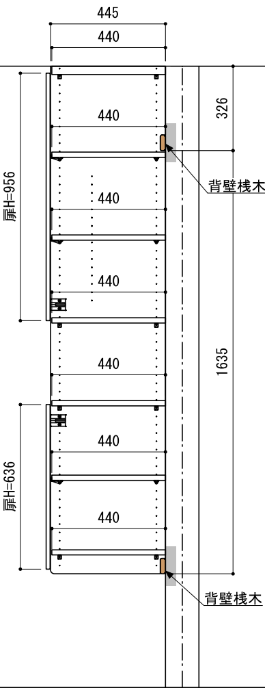
B-B' 断面
