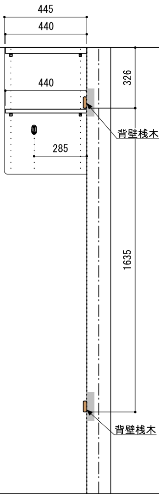
A-A' 断面
