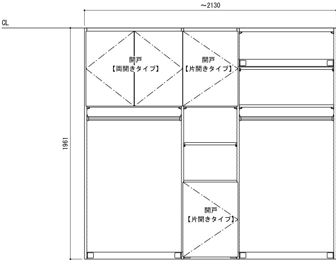
正面図（外観）
