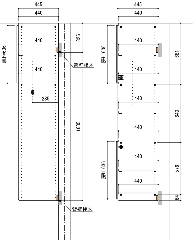
A-A' 断面
