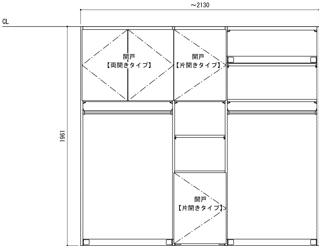
正面図（外観）
