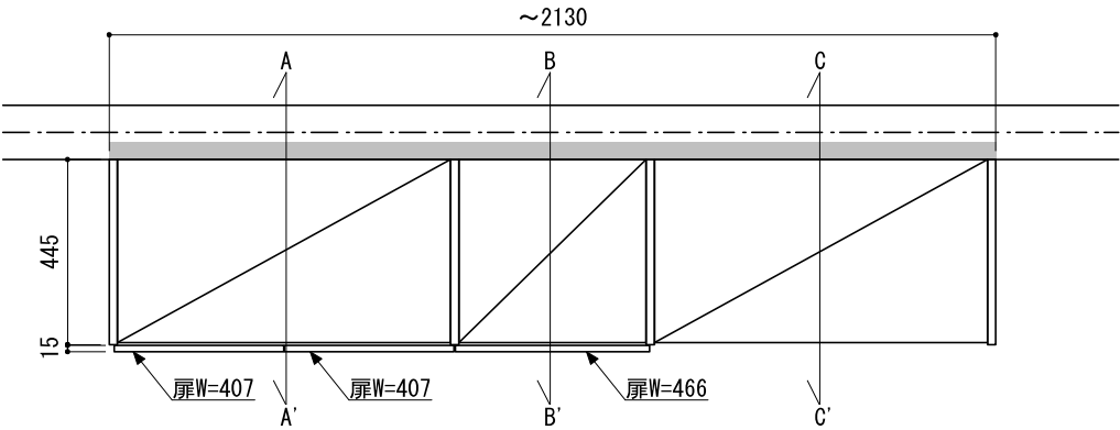
正面図（外観）
