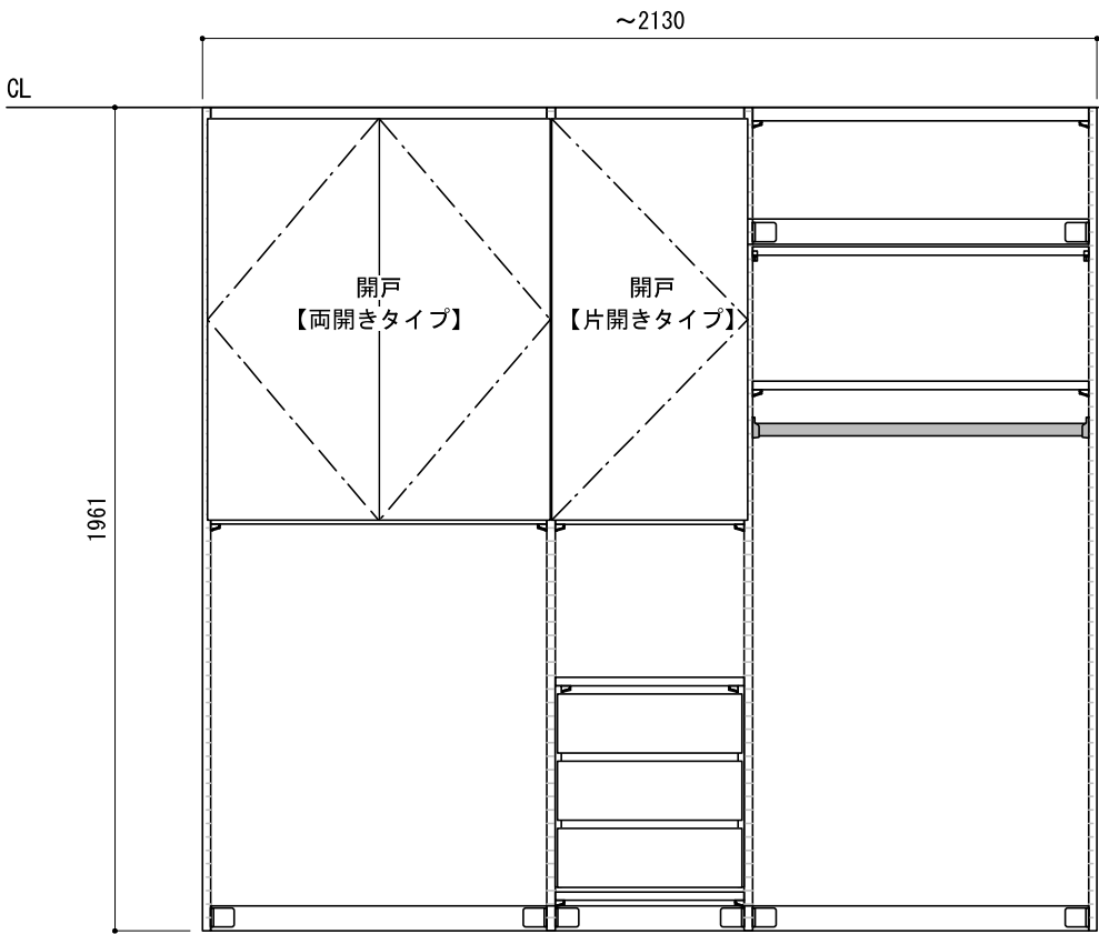
正面図（外観）
