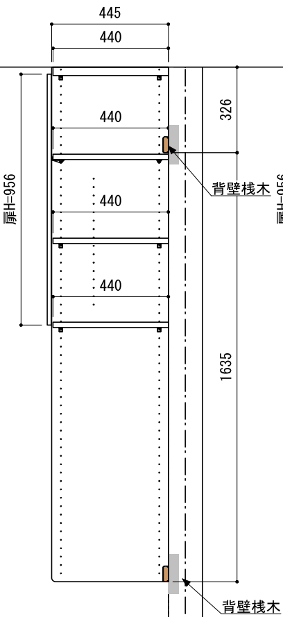
A-A' 断面
