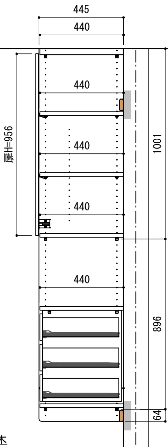
B-B' 断面
