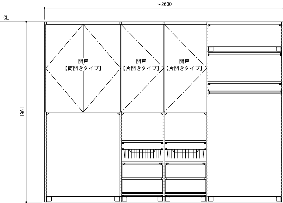
正面図（外観）
