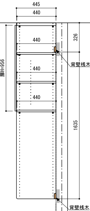
A-A' 断面
