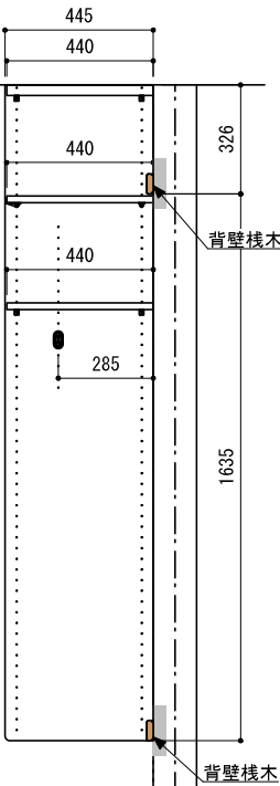
C-C' 断面
