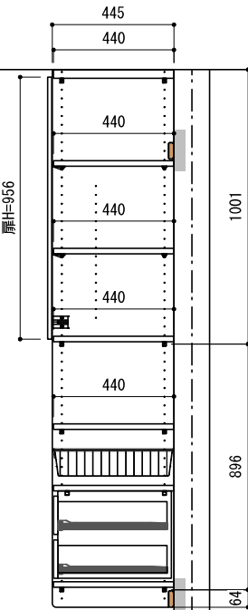
B-B' 断面
