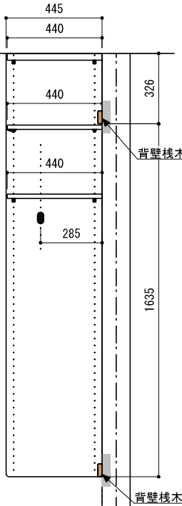
C-C' 断面
