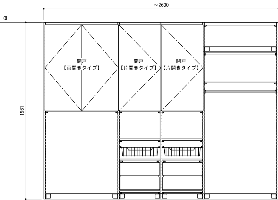
正面図（外観）
