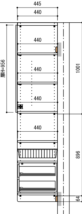
B-B' 断面
