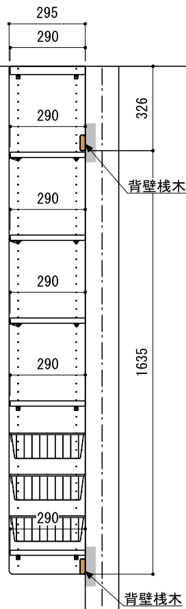
A-A' 断面
