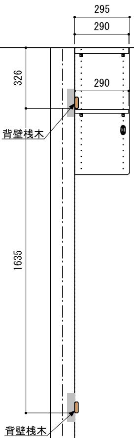
B-B' 断面
