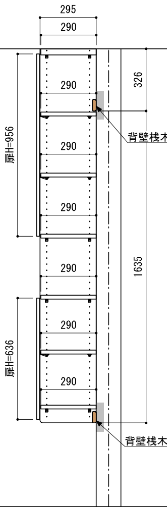
A-A' 断面
