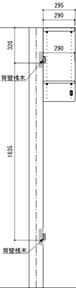
B-B' 断面
