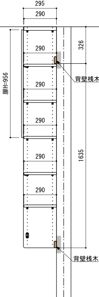
A-A' 断面
