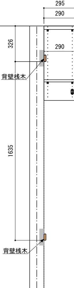
B-B' 断面
