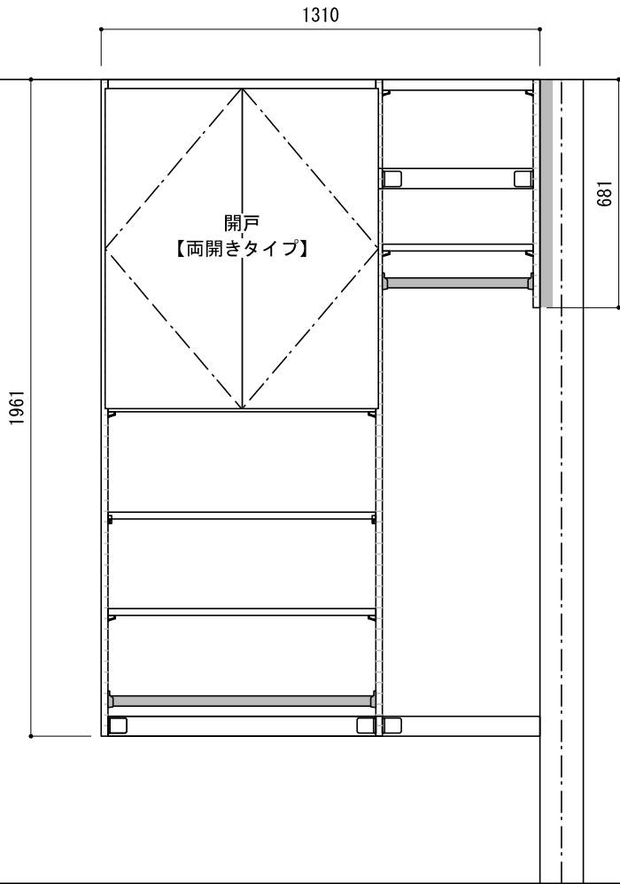
正面図（外観）
