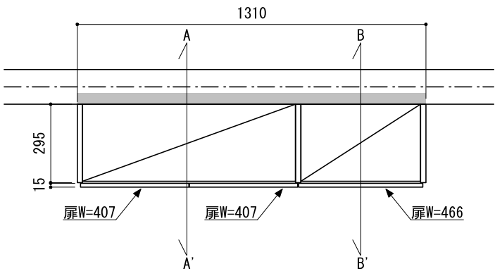
正面図（外観）
