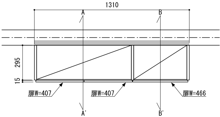
正面図（外観）
