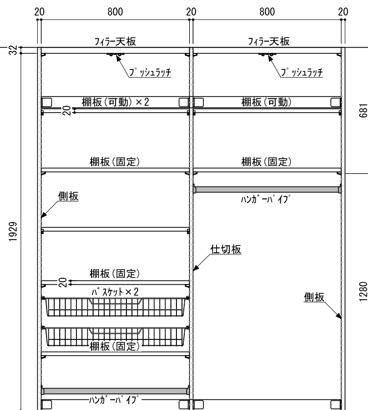
正面図（扉内部）
