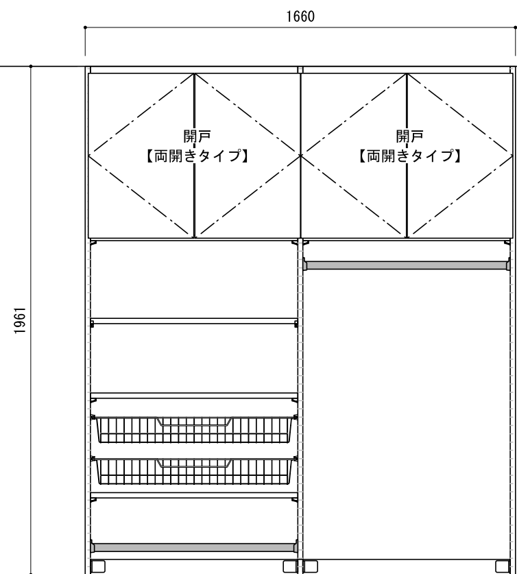
正面図（外観）
