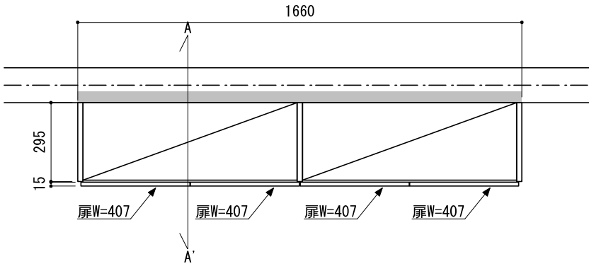
正面図（外観）
