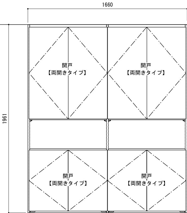
正面図（外観）
