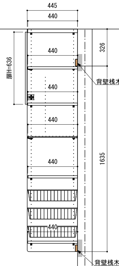
B-B' 断面
