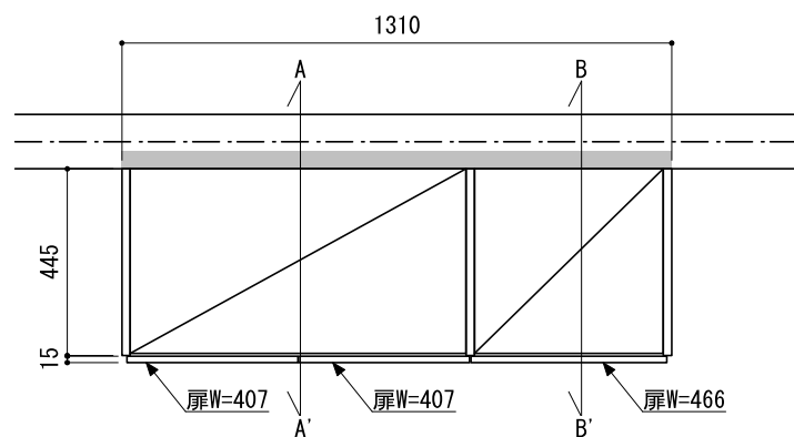
正面図（外観）
