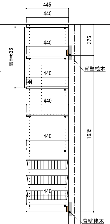
B-B' 断面
