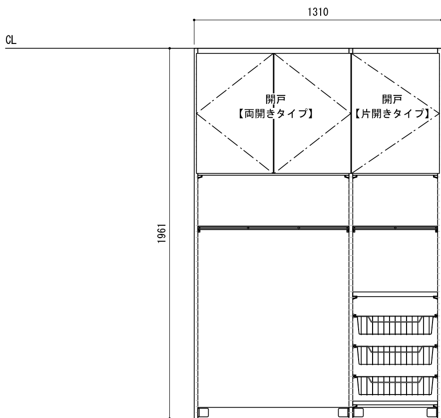
正面図（外観）
