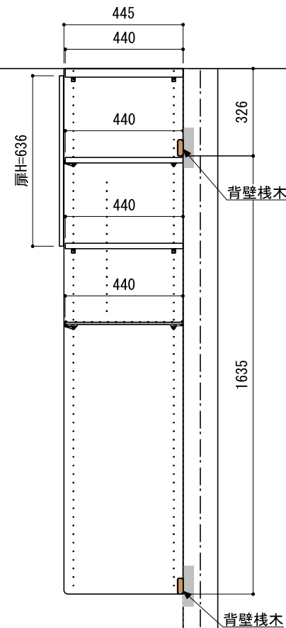
A-A' 断面
