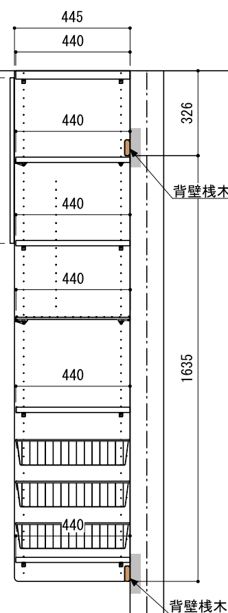
B-B' 断面
