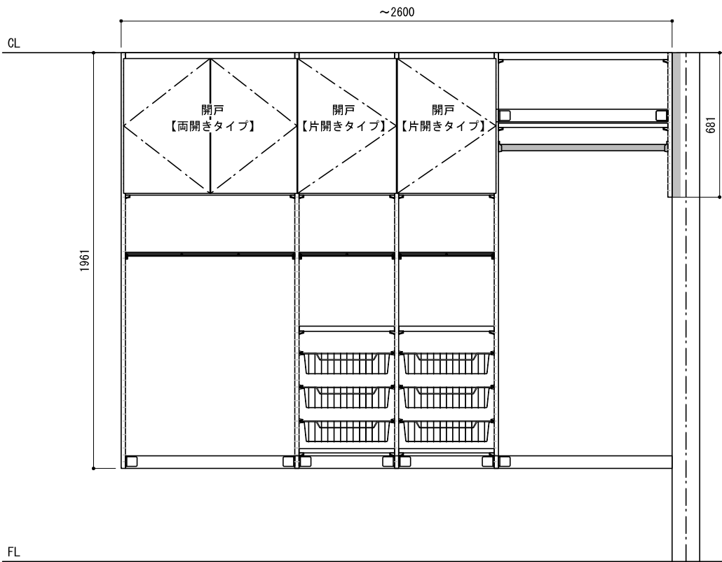
正面図（外観）
