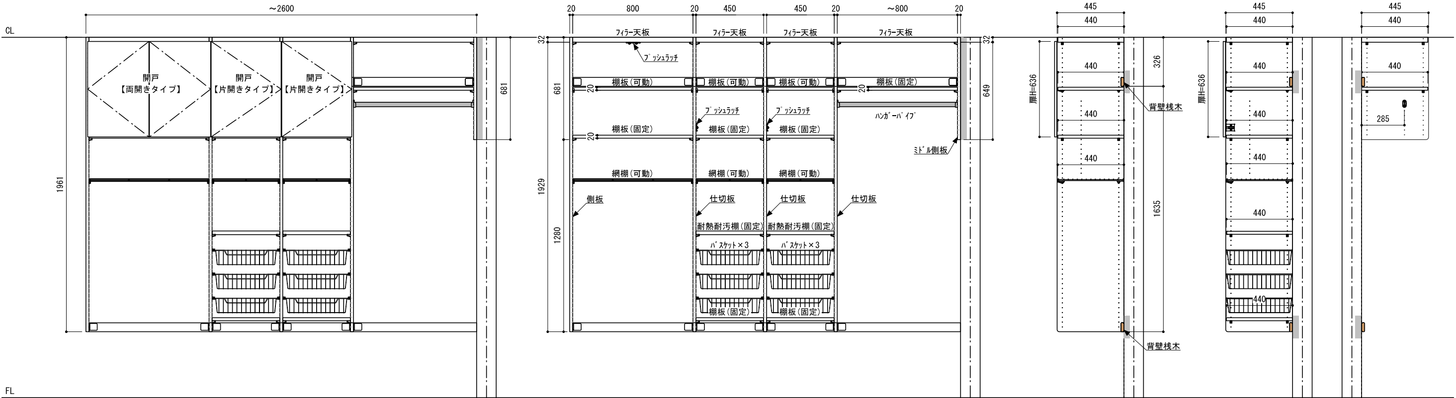
正面図（外観）
