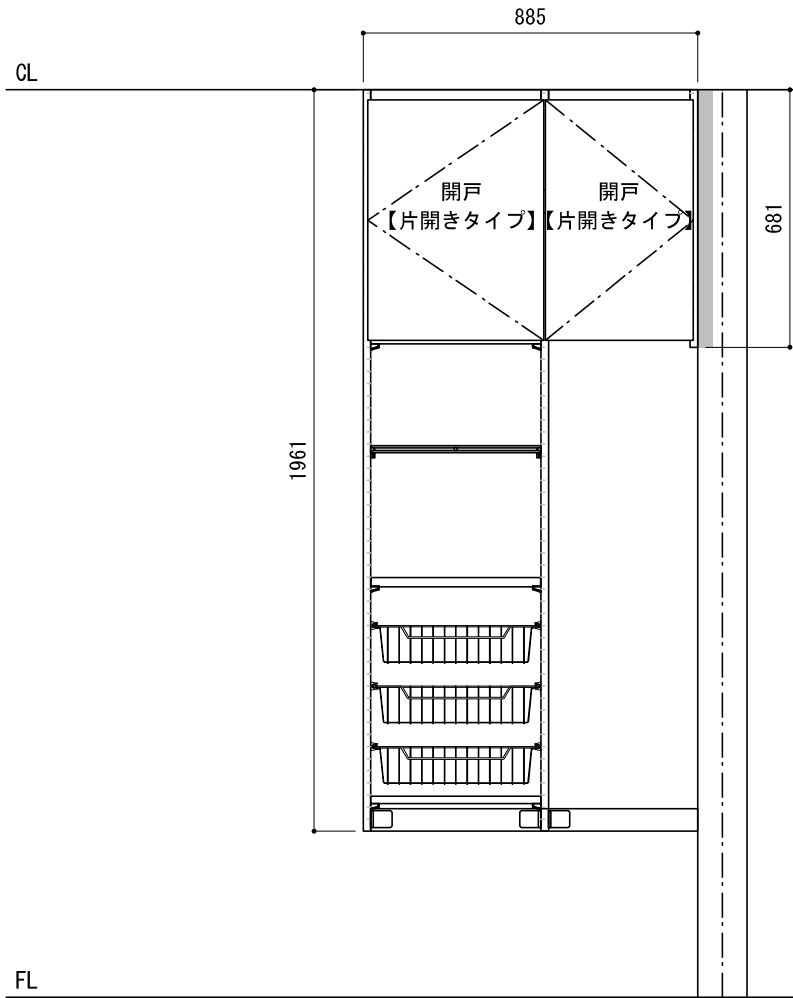
正面図（外観）
