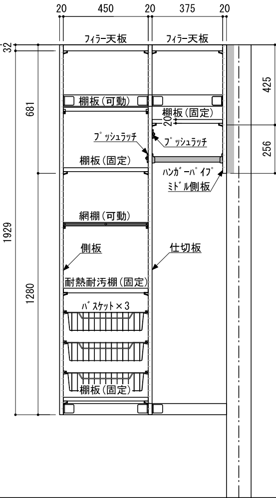
正面図（扉内部）
