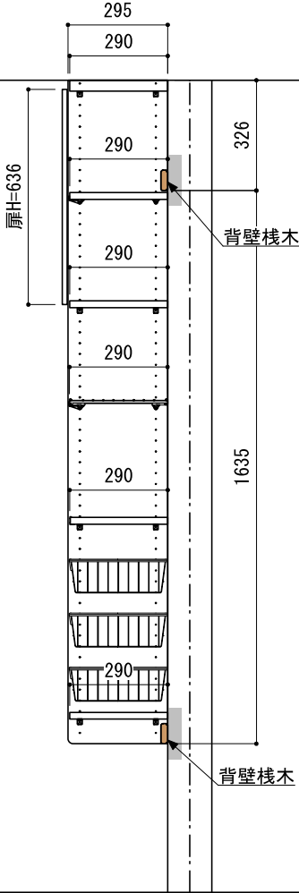
A-A' 断面
