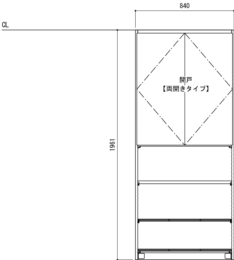
正面図（外観）
