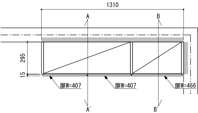
正面図（外観）
