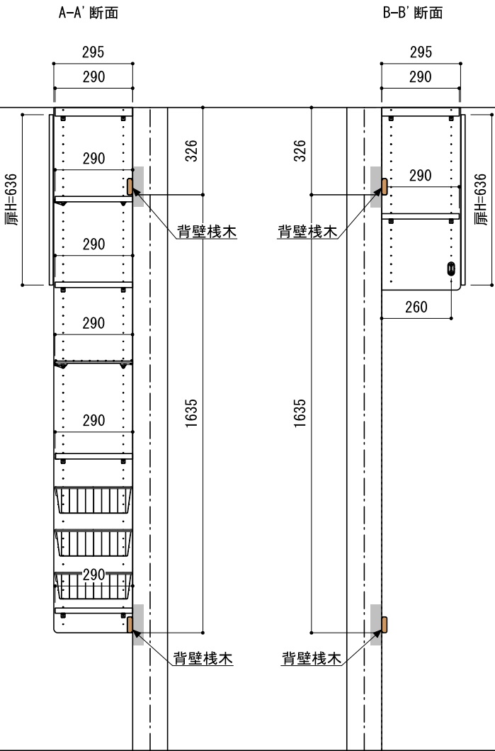
A-A' 断面
