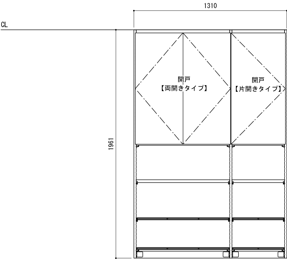
正面図（外観）
