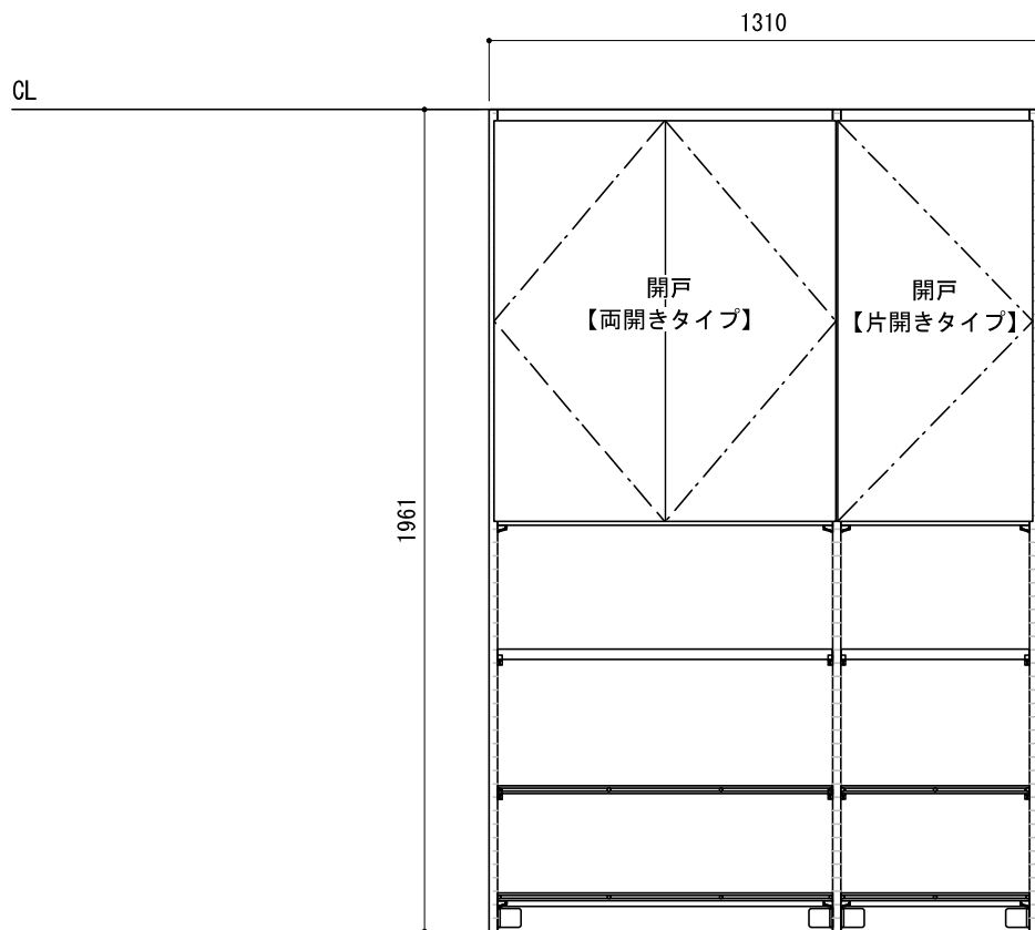
正面図（外観）
