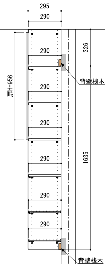
A-A' 断面
