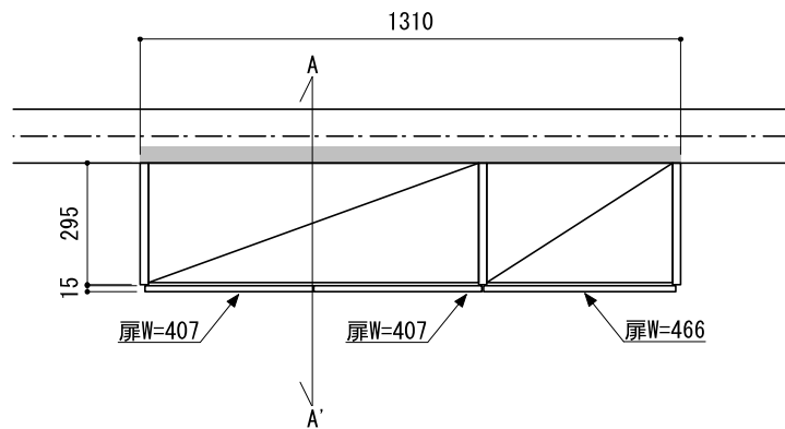
正面図（外観）
