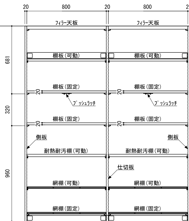
正面図（扉内部）
