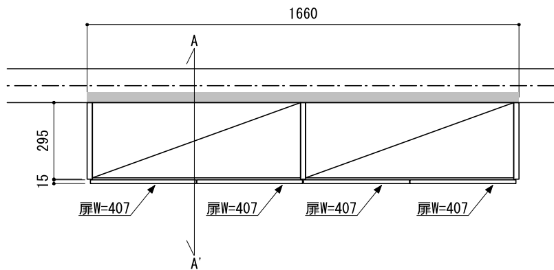
正面図（外観）
