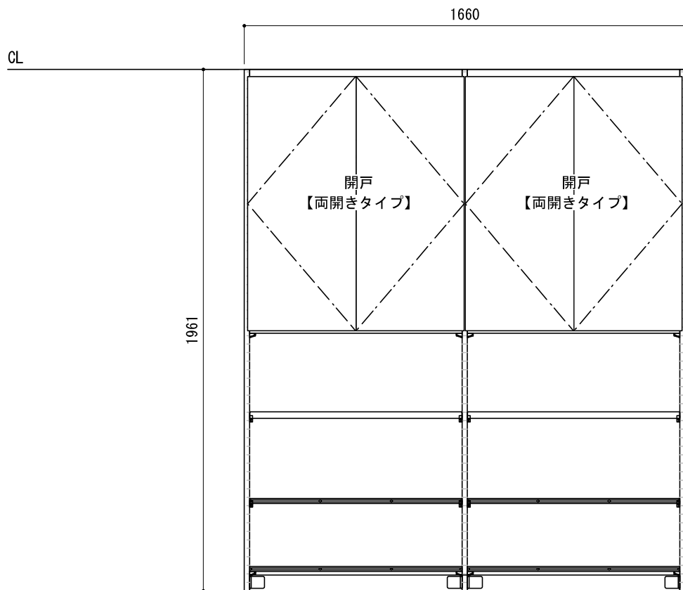
正面図（外観）
