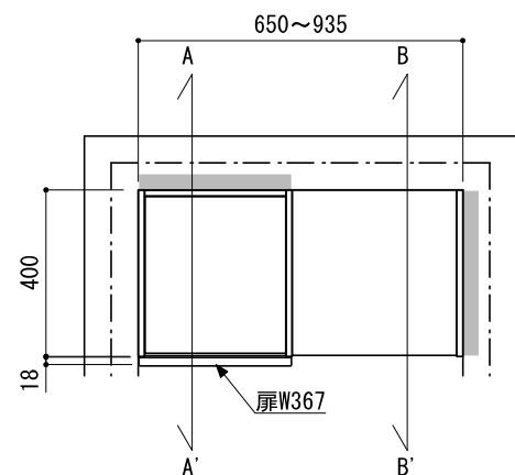
正面図（扉有り）
