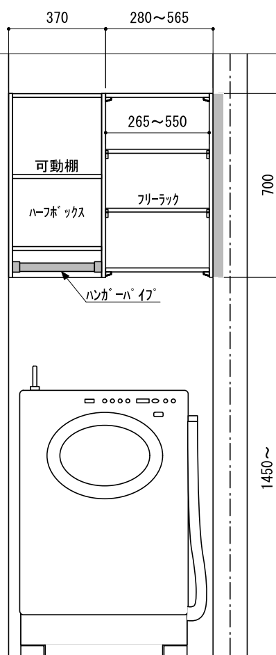
正面図（扉無し）
