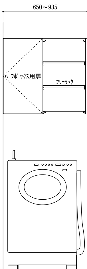
正面図（扉有り）
