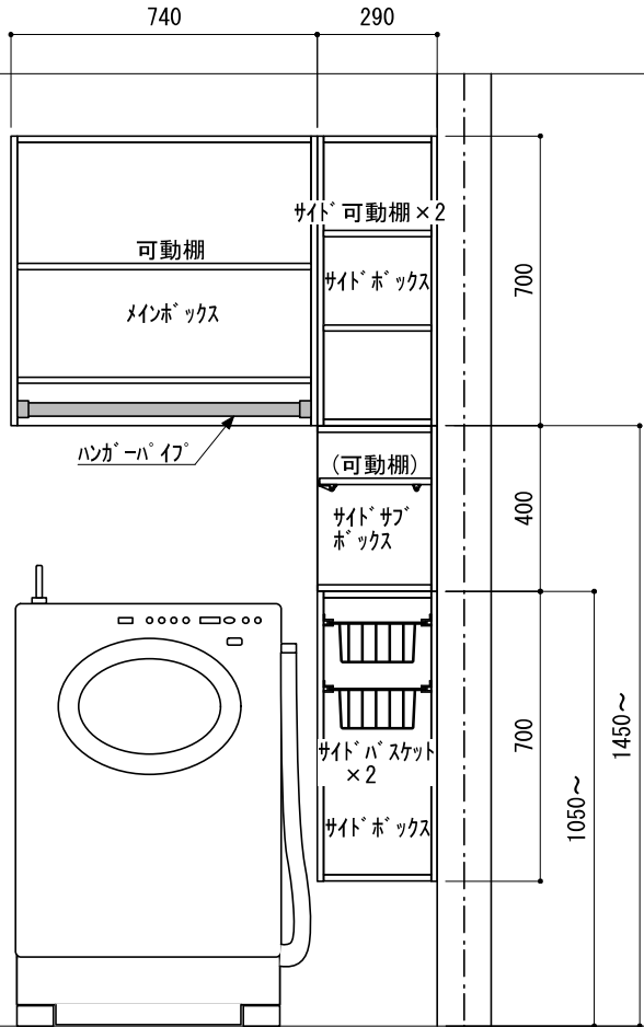
正面図（扉無し）
