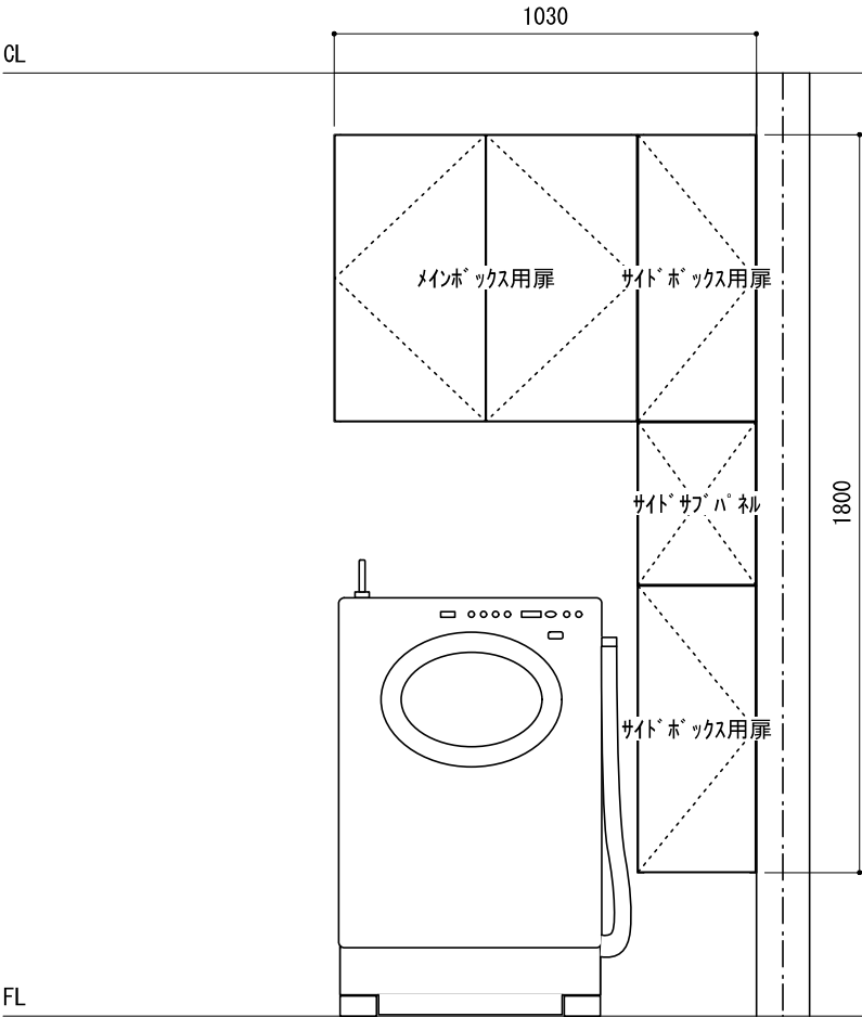
正面図（扉有り）
