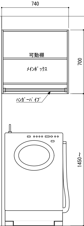
正面図（扉無し）
