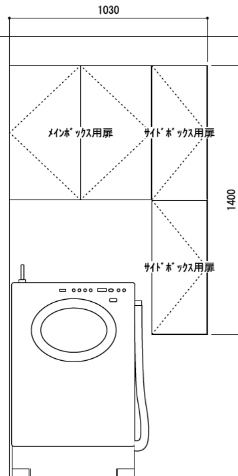
正面図（扉有り）
