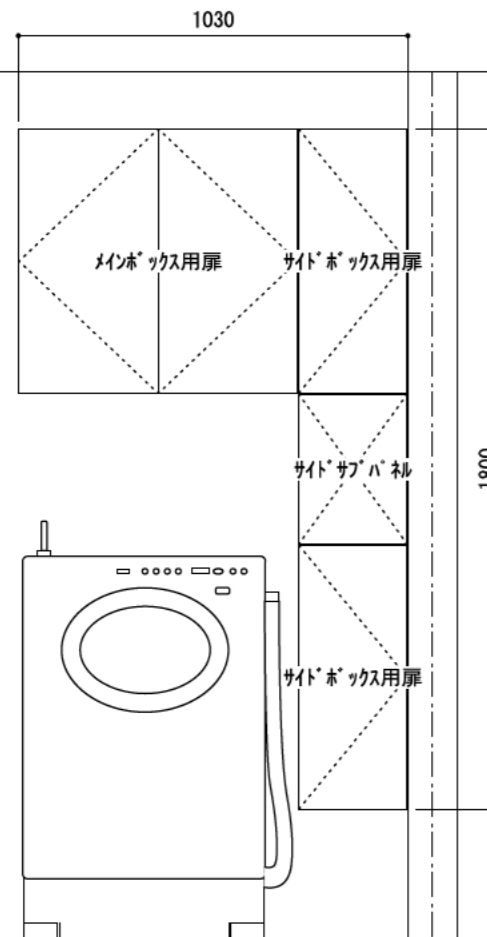
正面図（扉有り）
