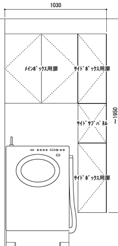
正面図（扉有り）
