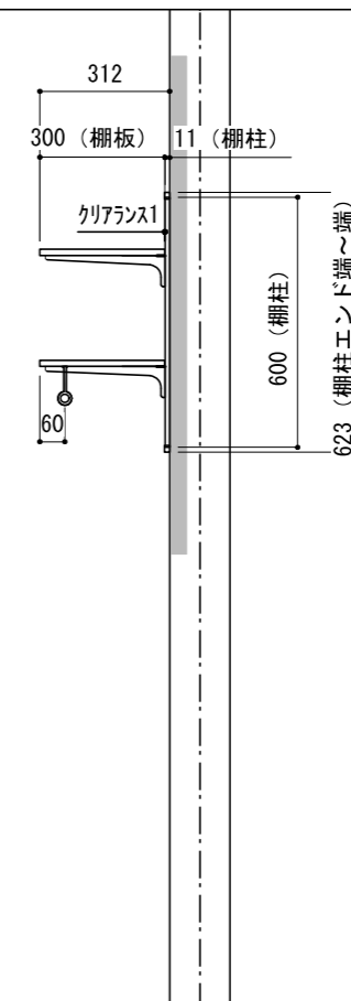
A-A' 断面
