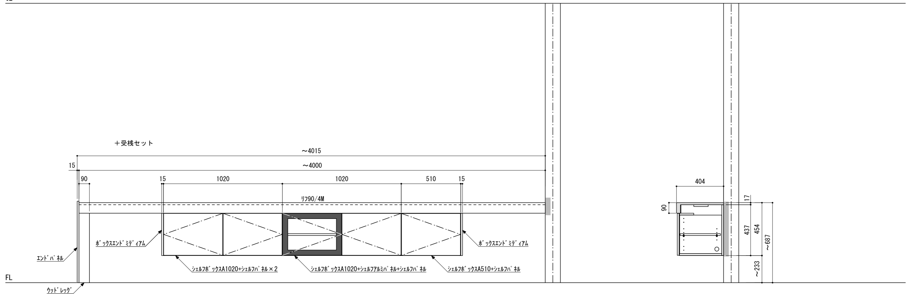
A-A' 断面
