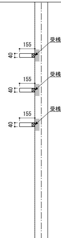
A-A' 断面
