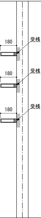
A-A' 断面
