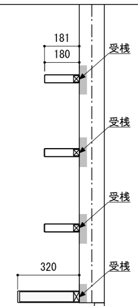
A-A' 断面
