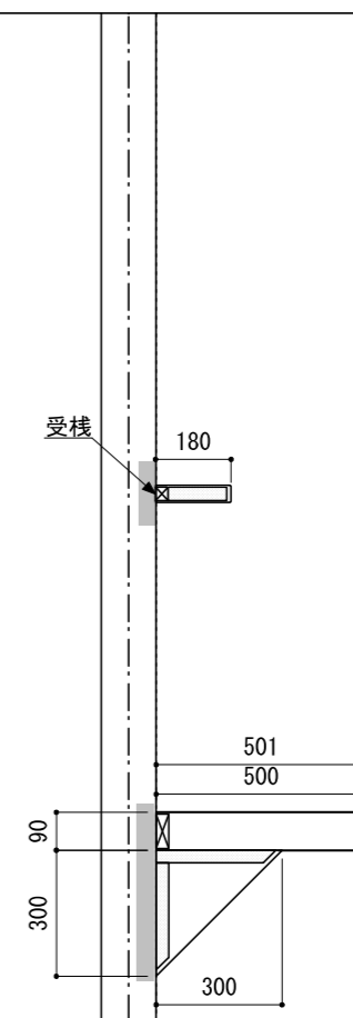
A-A' 断面
