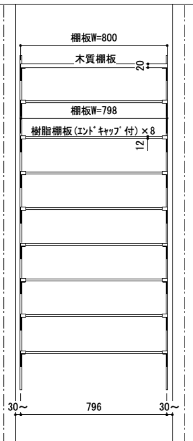
A 立面
