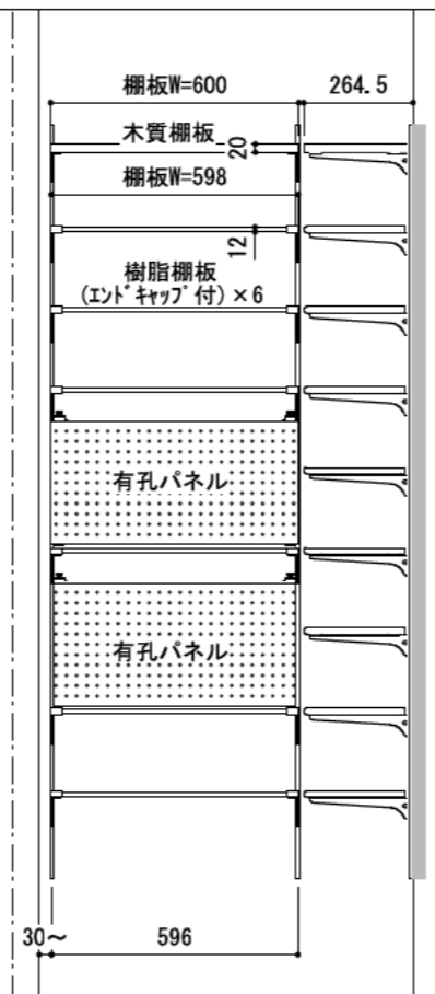
B 立面
