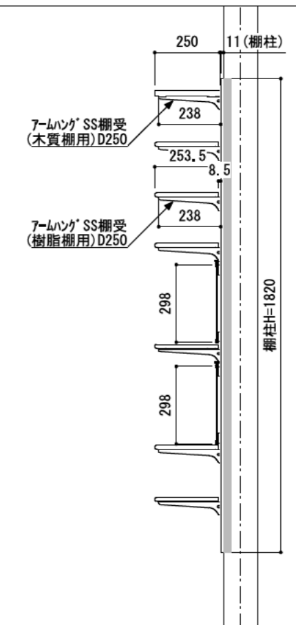
B-B' 断面
