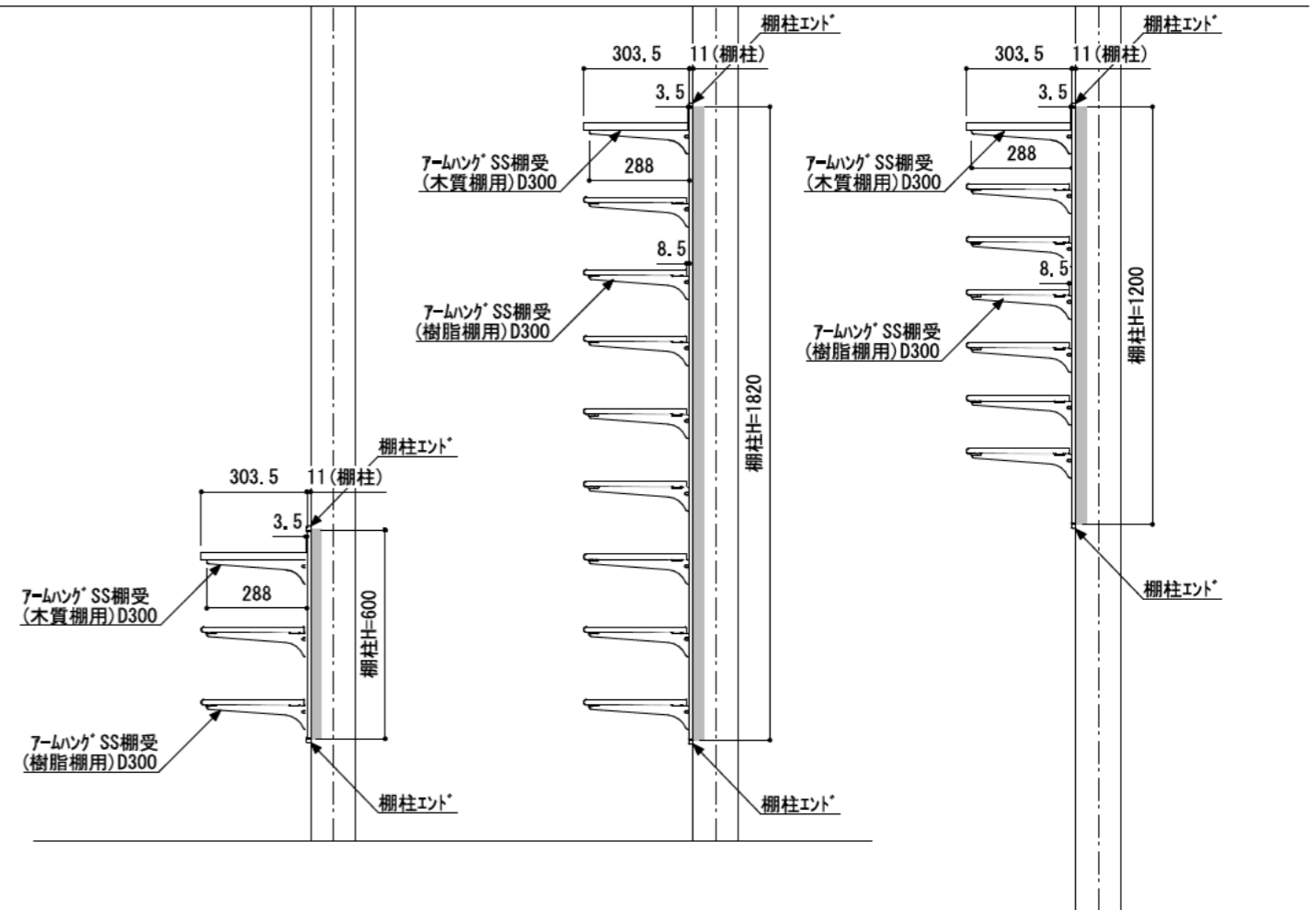
A-A' 断面
