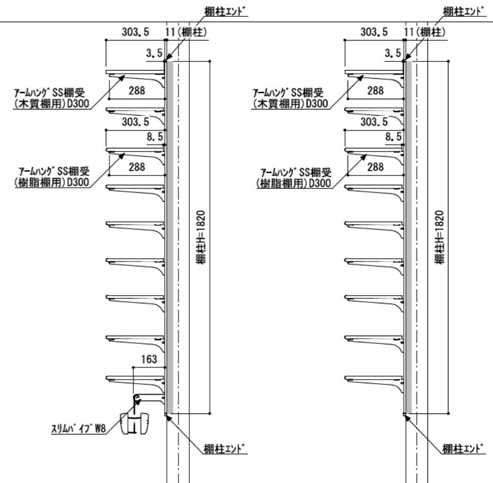
A-A' 断面
