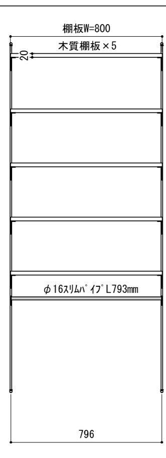
A立面
