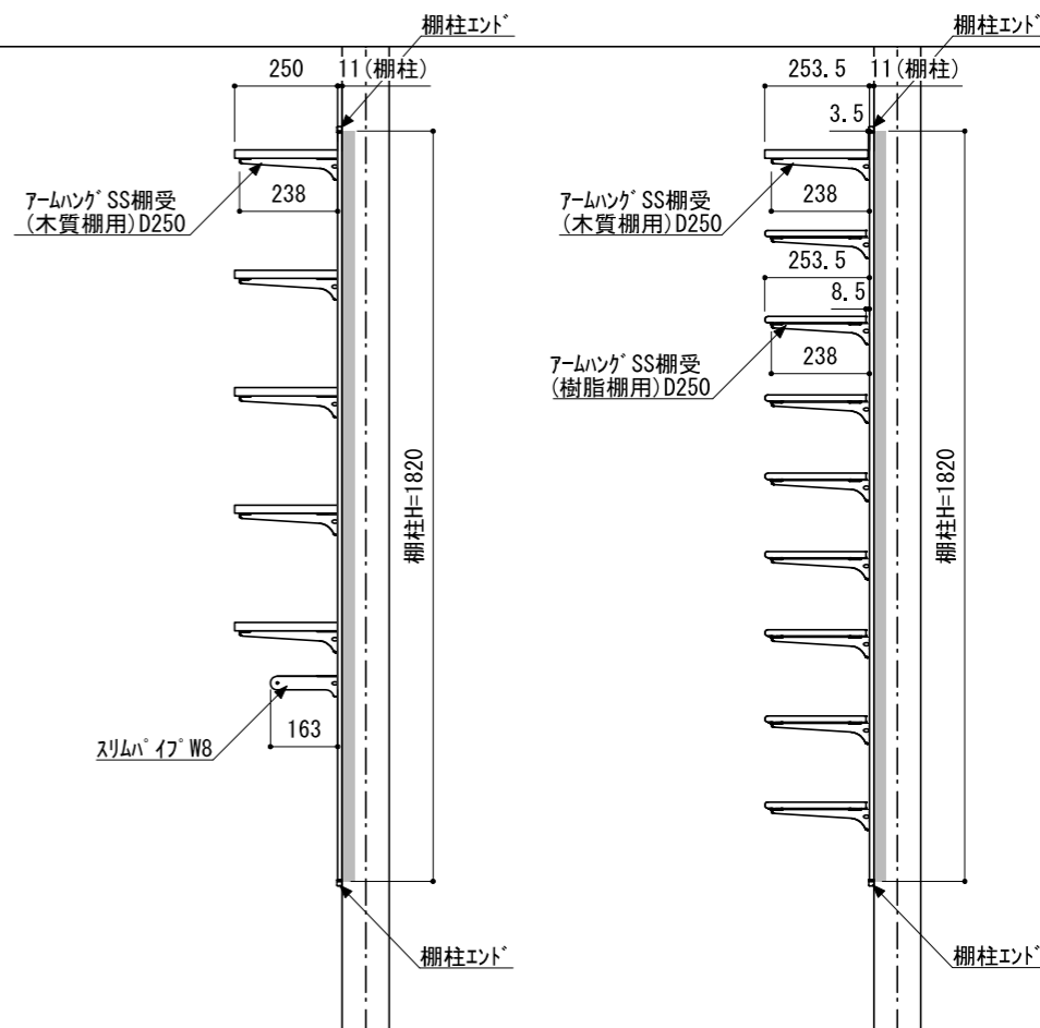
A-A' 断面
