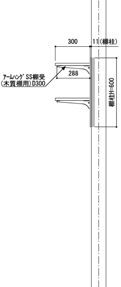
A-A' 断面
