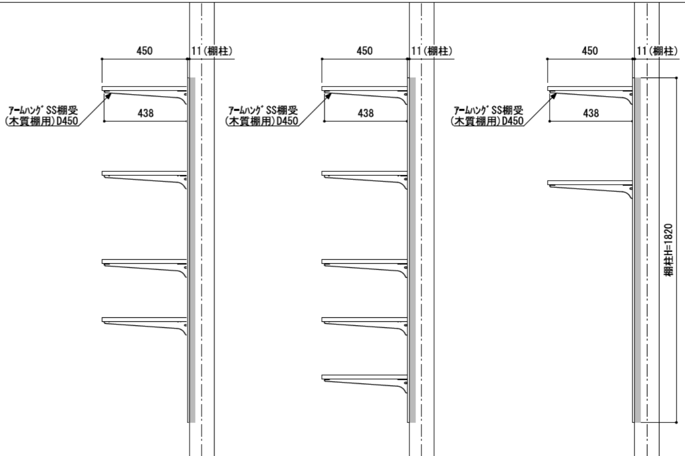
A-A' 断面
