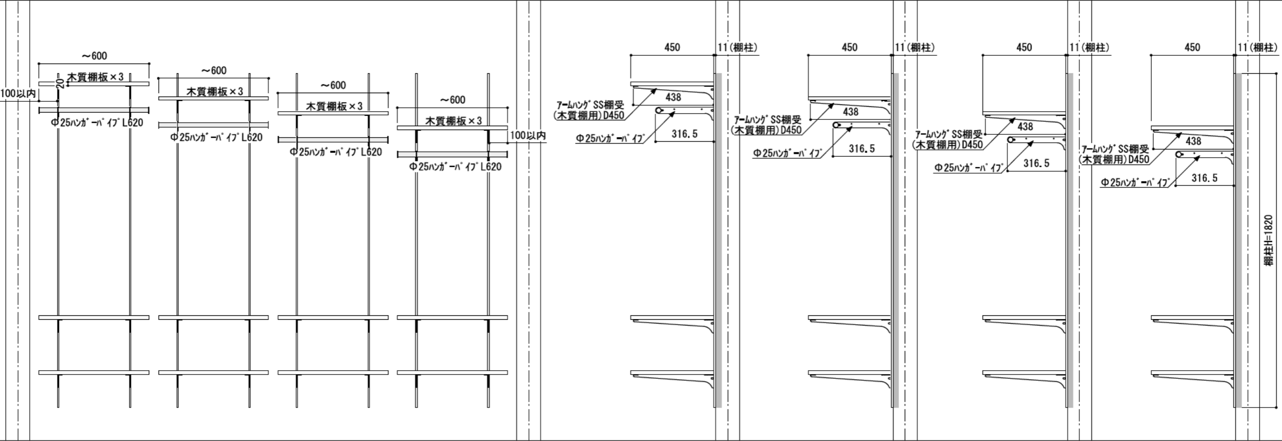
A-A' 断面
