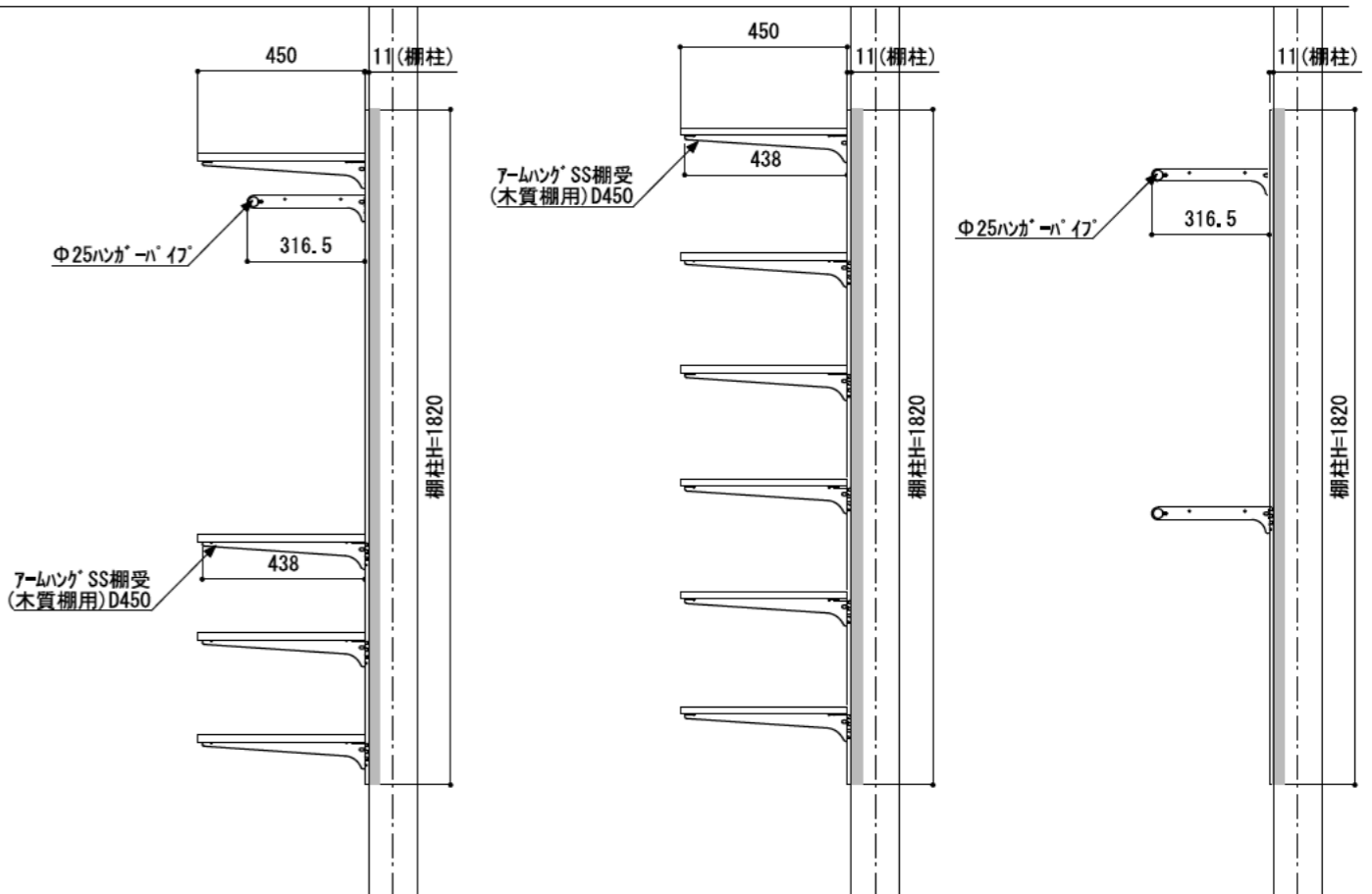
A-A' 断面
