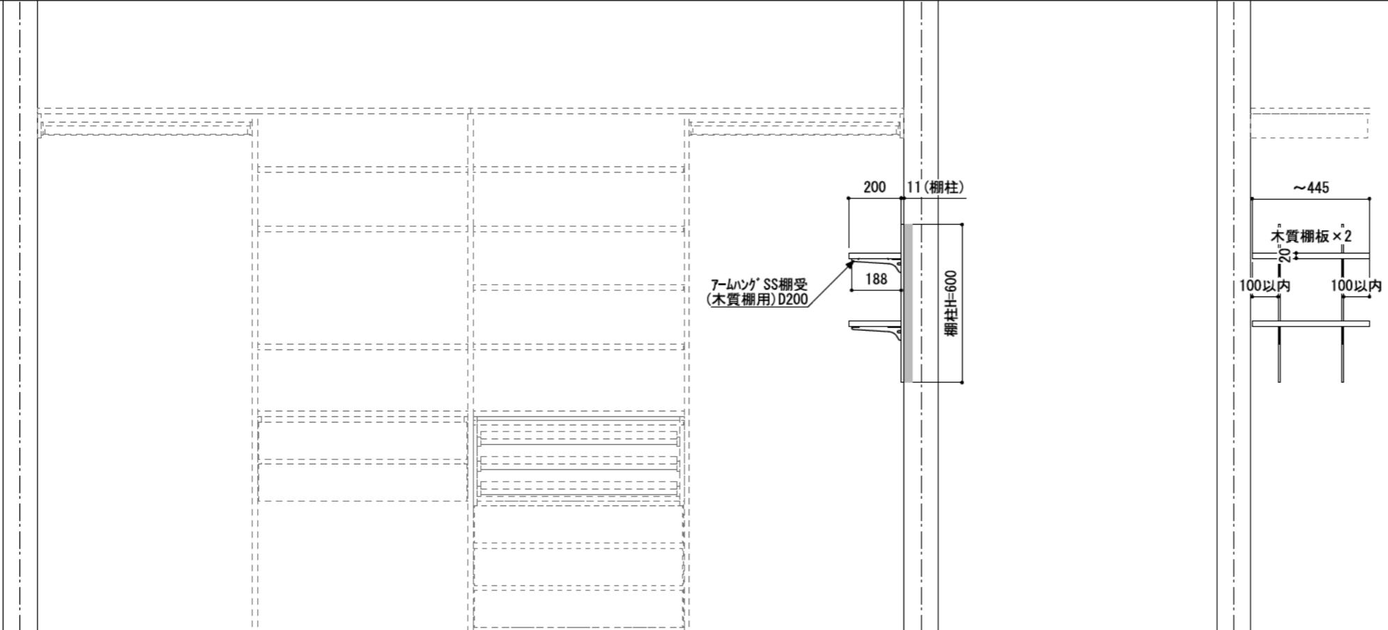
A-A' 断面
