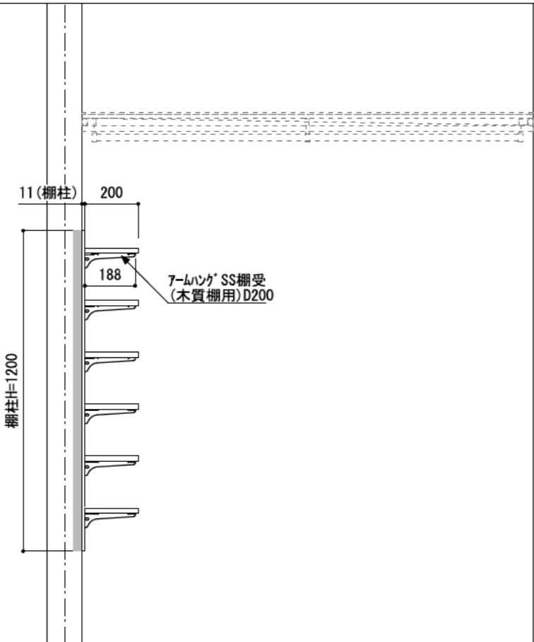
A-A' 断面
