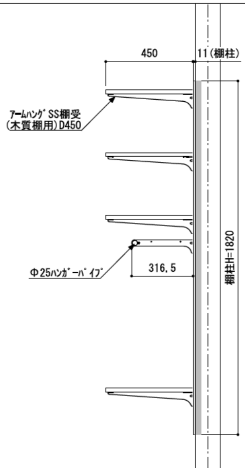
B-B' 断面
